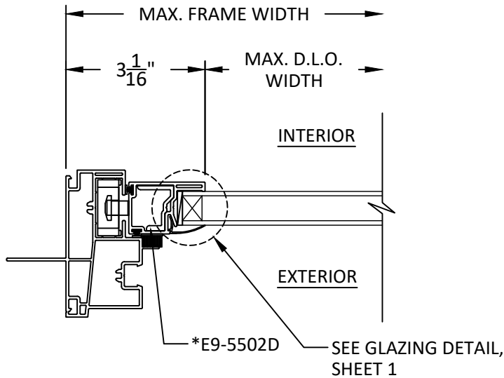
F 6 HORIZONTAL SECTION VENT LEFT JAMB
