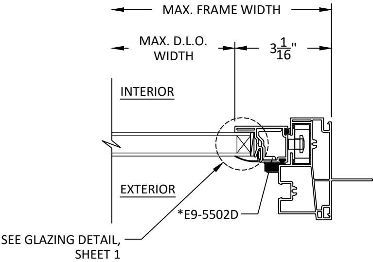
G 6 HORIZONTAL SECTION VENT RIGHT JAMB
