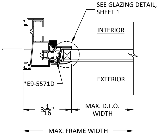
D 6 HORIZONTAL SECTION FIXED LEFT JAMB
